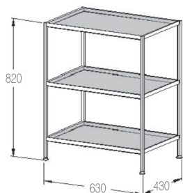
Столик для инструментов ИС-1 ; 17,85 кг
