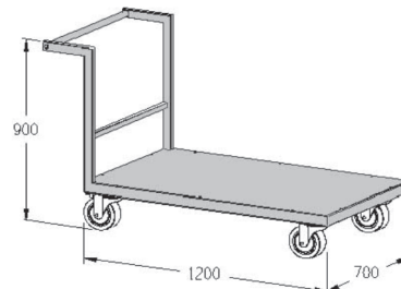
ТК-40 (до 300 кг); 38,3 кг
