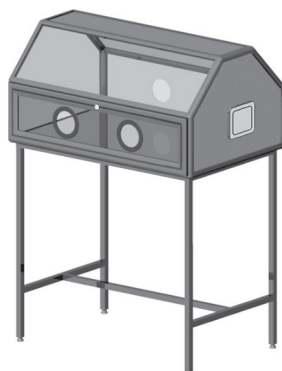
Бокс стерильный 42,88 кг
